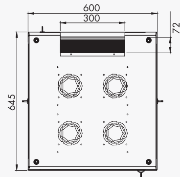
Üst görünüş
