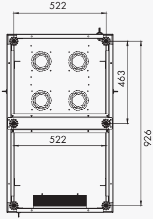
Alt görünüş*
