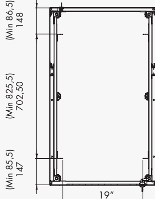
Kabinet cihaz dikme yerleşimi
