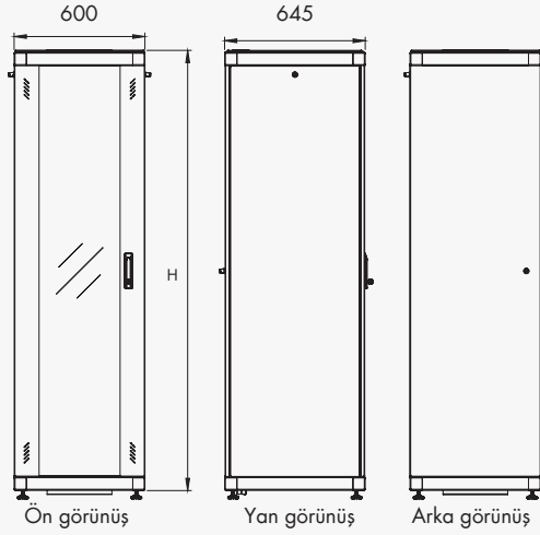
Ön görünüş
