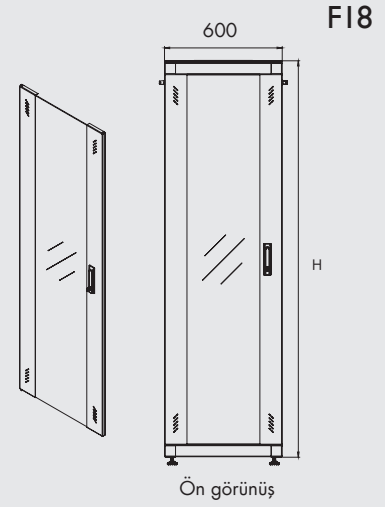
Ön görünüş
