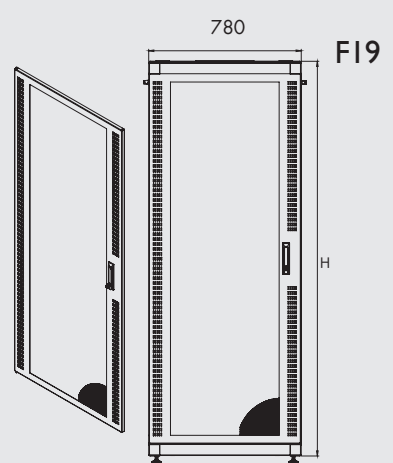
Ön görünüş
