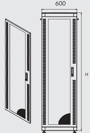
Ön görünüş
