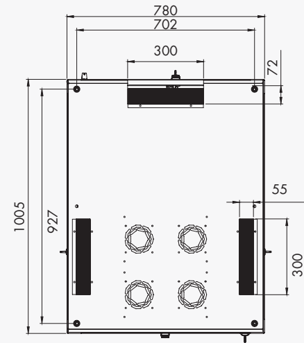
Üst görünüş
