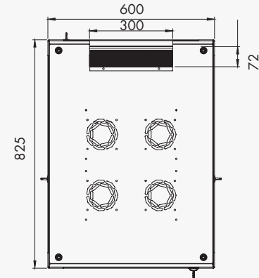
Üst görünüş
