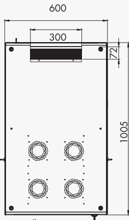
Üst görünüş
