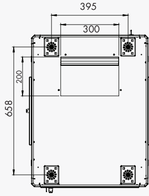
Alt görünüş
