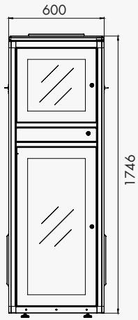
Ön görünüş
