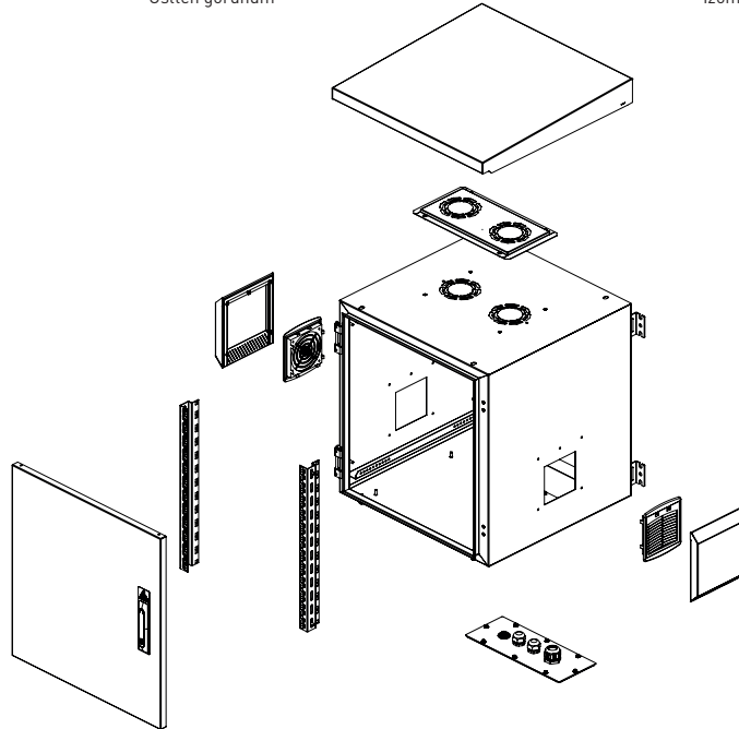
Patlatılmış görünüm
