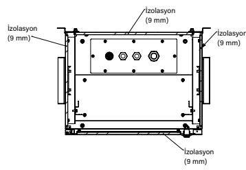
Yandan görünüm
