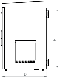
Yandan görünüm
