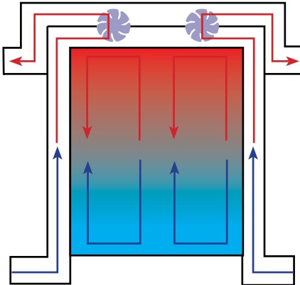
Hava sirkülasyon şeması
