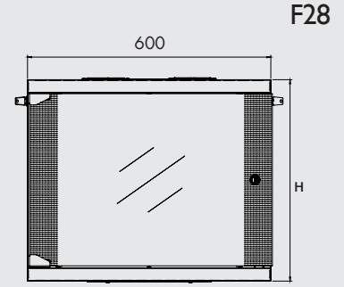
Ön görünüş
