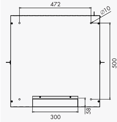
Alt görünüş
