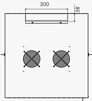
Üst görünüş
