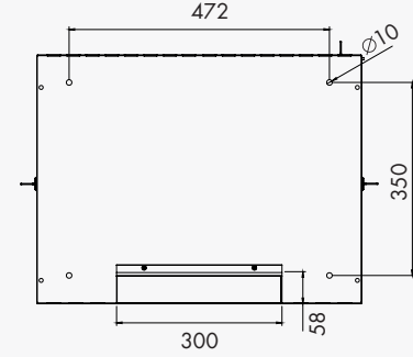
Alt görünüş
