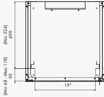
Kabinet cihaz dikme yerleşimi
