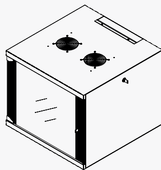
İzometrik görünüş
